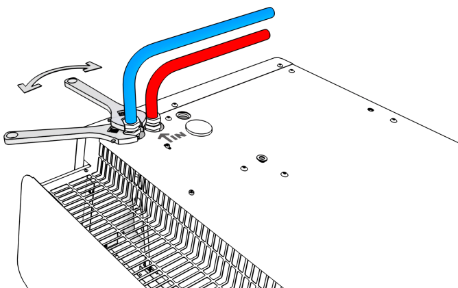
RYS. 10.3 KONTROWANIE.
