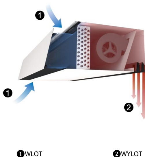
RYS. 2.1 KIERUNEK PRZEPŁYWU POWIETRZA.
