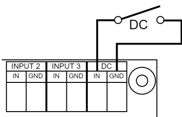
RYC. 9.3 PODŁĄCZENIE CZUJNIKA DRZWIOWEGO.
