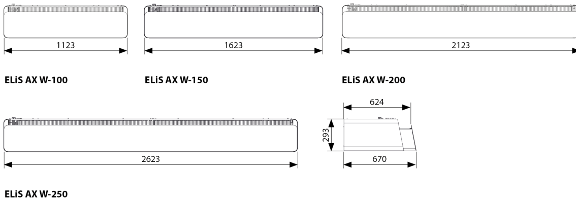
RYS. 4.1 PODSTAWOWE WYMIARY.
