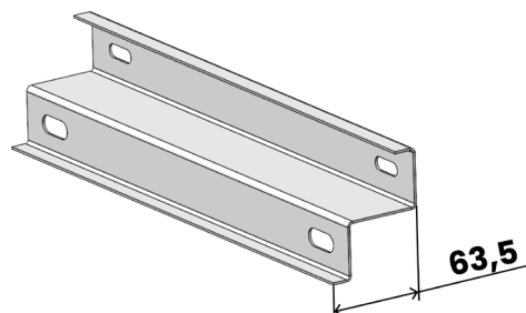
RYS. 7.6. SZEROKOŚĆ WSPORNIKA BOCZNEGO
