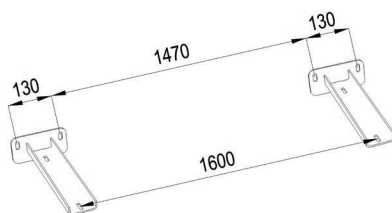
RYS. 6.4 ODLEGŁOŚCI WSPORNIKÓW DLA ELIS AX W 200.
