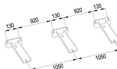
RYS. 6.5 ODLEGŁOŚCI WSPORNIKÓW DLA ELIS AX W 250.
