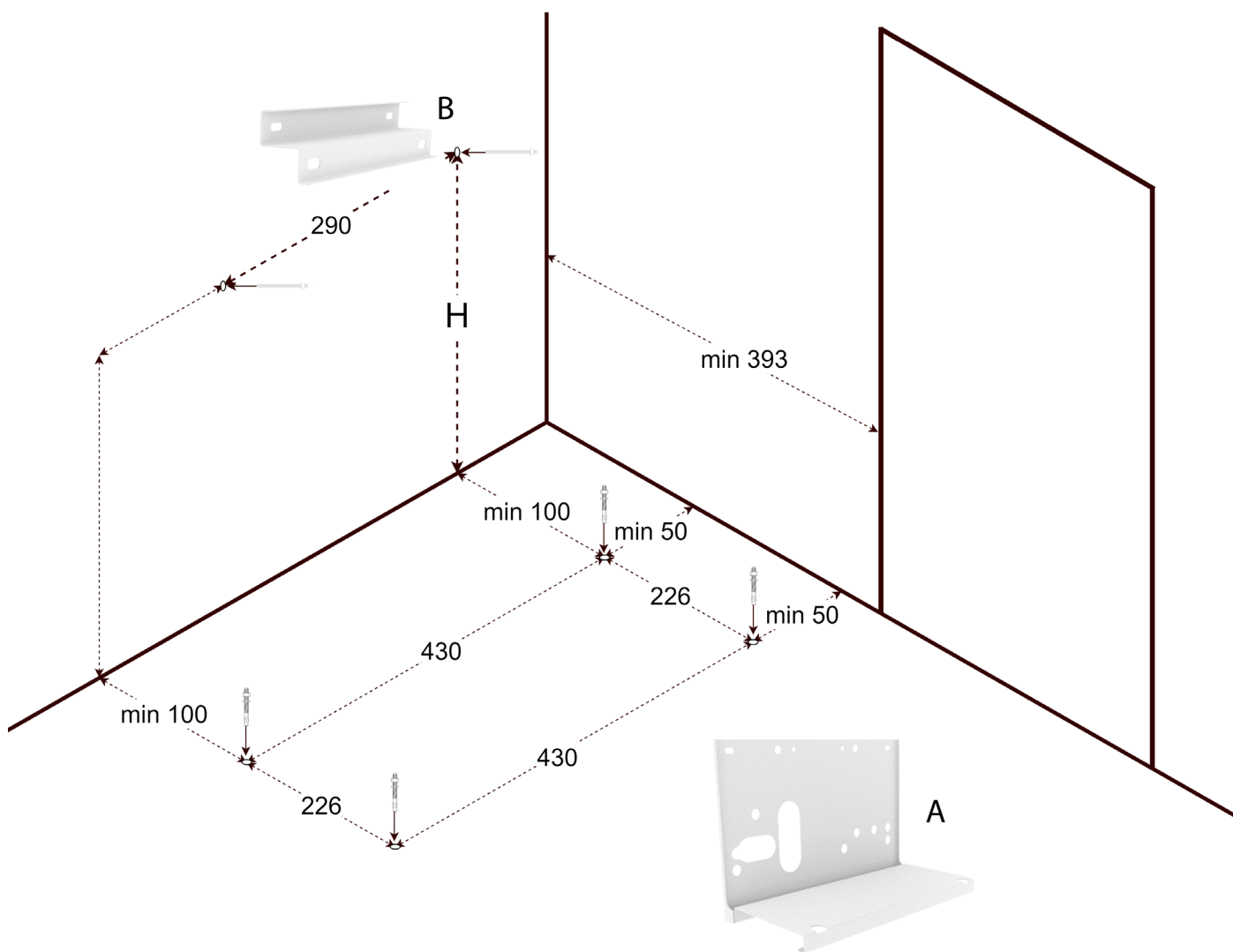
RYS. 7.4. SCHEMAT UMIEJSCOWIENIA OTWORÓW MONTAŻOWYCH PODSTAWY (A) I WSPORNIKA BOCZNEGO (B).
