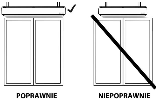
RYS. 5.1 MONTAŻ POZIOMY.
