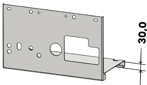
RYS. 7.5. WYSOKOŚĆ PODSTAWY
