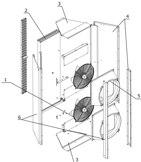
РИС. 3.1 СТРОИТЕЛЬСТВО ELiS G N/W/E.
