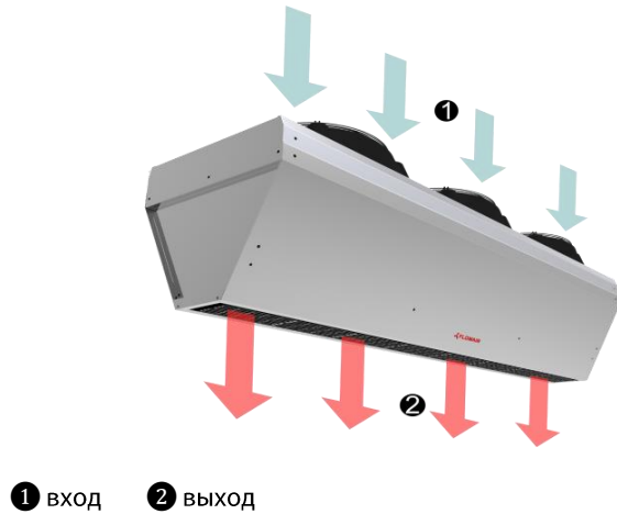
РИС. 2.1 НАПРАВЛЕНИЕ ВОЗДУШНОГО ПОТОКА.
