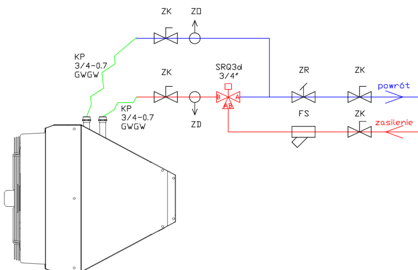
РYS.16.1. ПРИМЕР СОЕДИНЕНИЯ ГИДРАВЛИЧЕСКИХ КОМПОНЕНТОВ. Параметр
