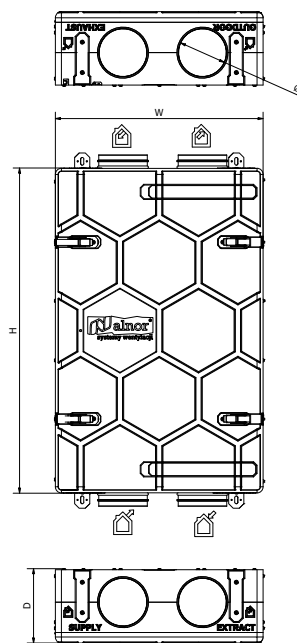
HRU-SlimAIR
